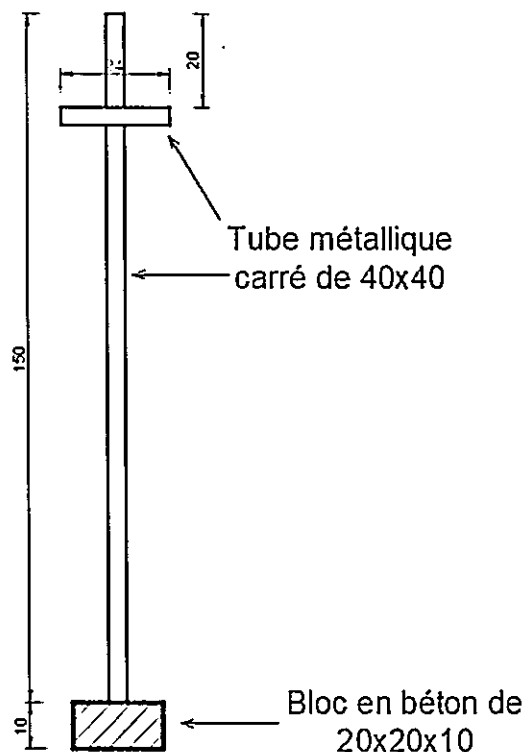
Figure 1: schéma de la dame manuelle
